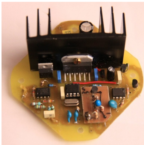
Ancien circuit de puissance, utilisant un C.I. de commande de moteur, nécessitant un radiateur
