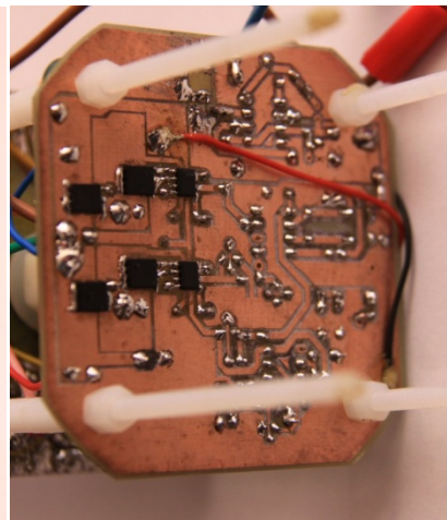
Nouveau circuit de puissance, à transistors MOSFET de très faible R_{DS(on)} , en CMS, sans radiateur
